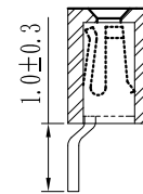
PCB板示意图
